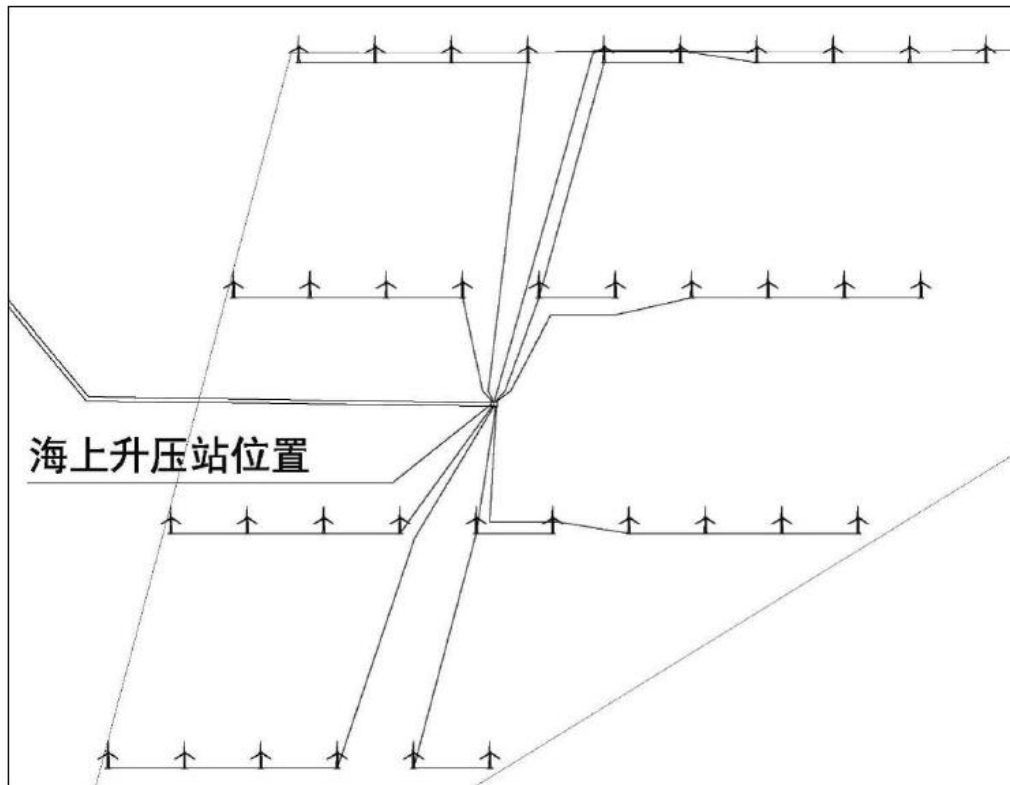
图 3.5-5 方案二路由布置图
