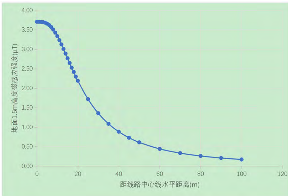
图 5.8-6 线路磁场强度变化趋势图
