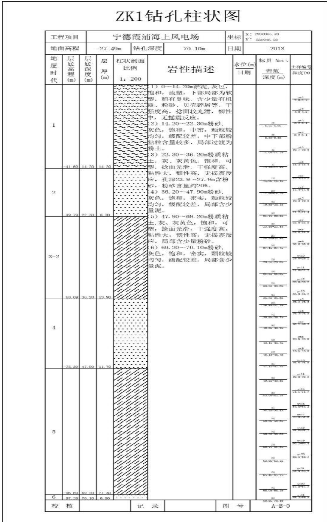
图 4.1-2 ZK1 钻孔柱状图
