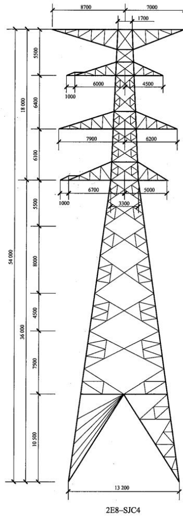
图 5.8-4 本预测选取典型杆塔图
