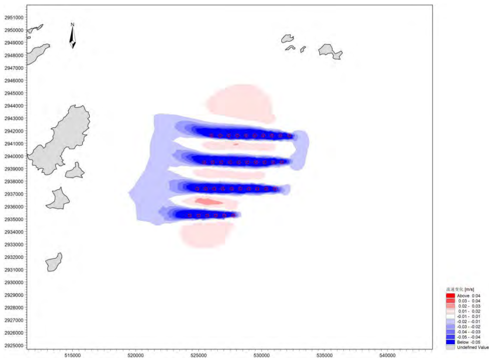
图 5.1-18 工程前后大潮涨急流速变化 (单位: m/s)
