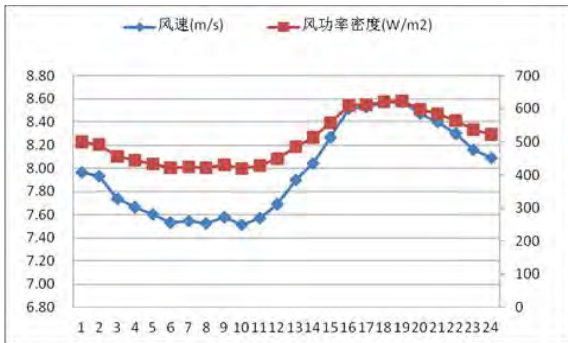
图 4.2-4 测风塔 80m 高度逐时平均风速及风功率密度变化曲线
