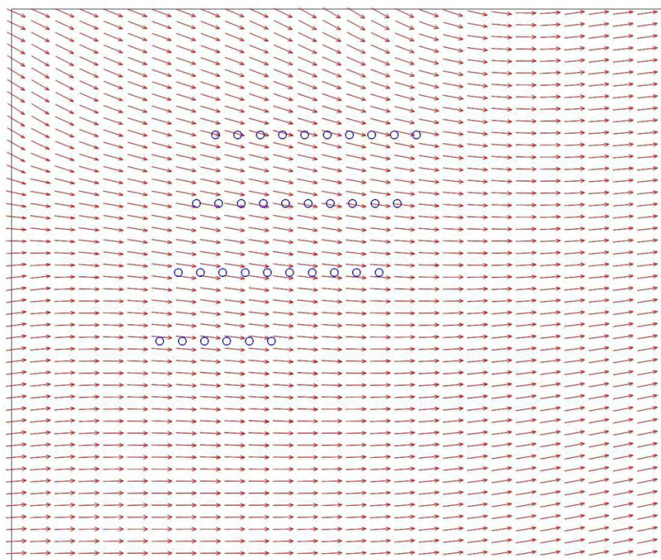
图 5.1-17 大潮期风电场附近海域落急时刻潮流场变化图 (黑色流矢：工程前；红色流矢：工程后)
