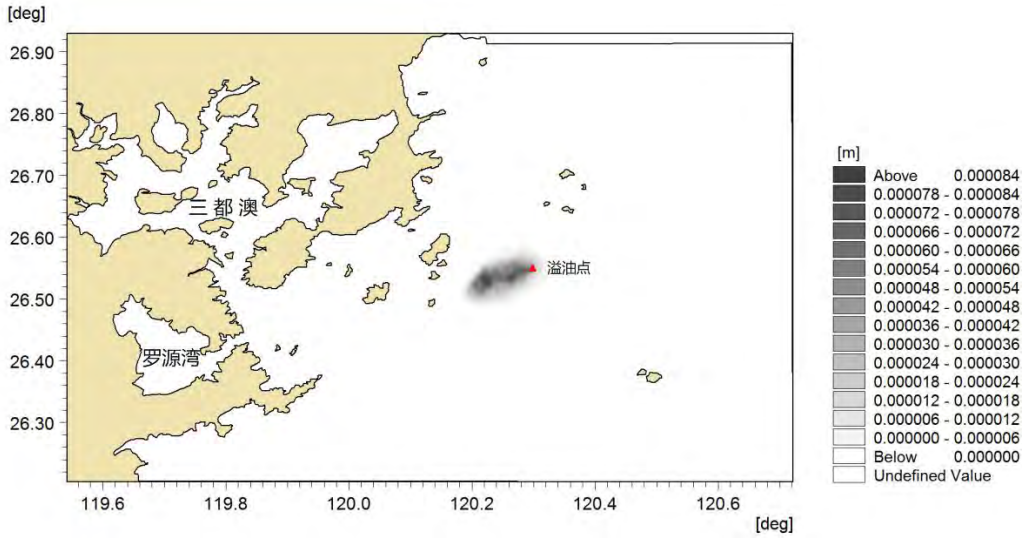
图 6.2-5 SE 低潮时溢油发生 72h 内最大影响范围图（单位：油膜厚度 m）
