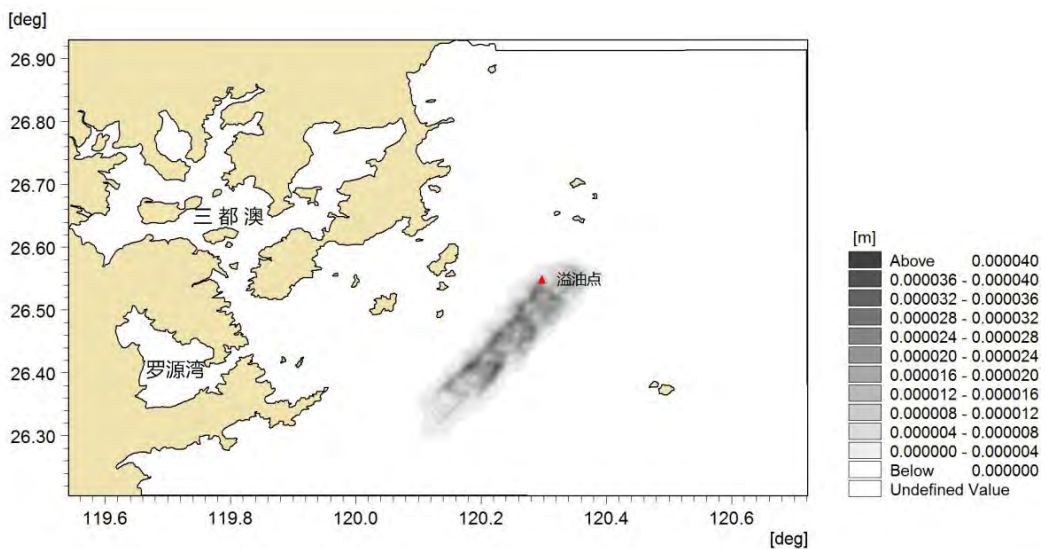
图 6.2-4 NNE 高潮时溢油发生 72h 内最大影响范围图（单位：油膜厚度 m）
