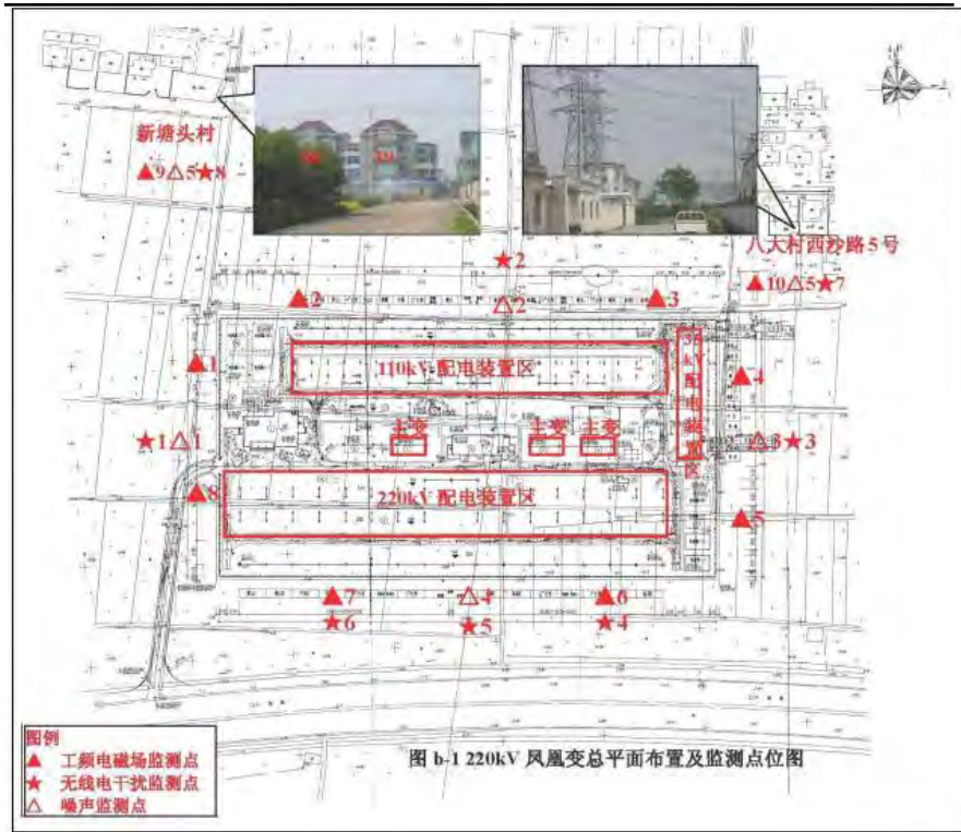
图 5.8-2 凤凰变电站总平面布置及监测点位图
