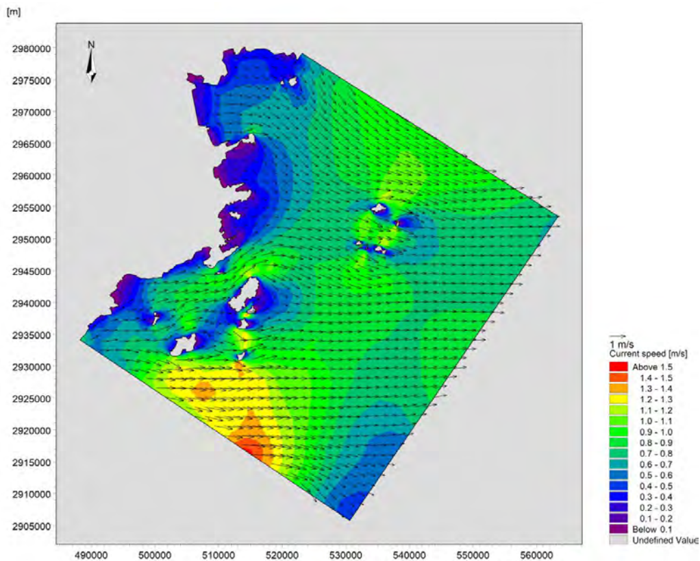
图 5.1-13 大潮期计算海域落急时刻潮流场（工程前）
