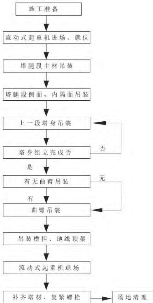
图 3.1-13 吊车吊装分解组塔施工工艺流程图
