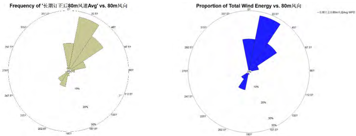
图 4.2-7 测风塔 80m 高度全年风向风能玫瑰图
