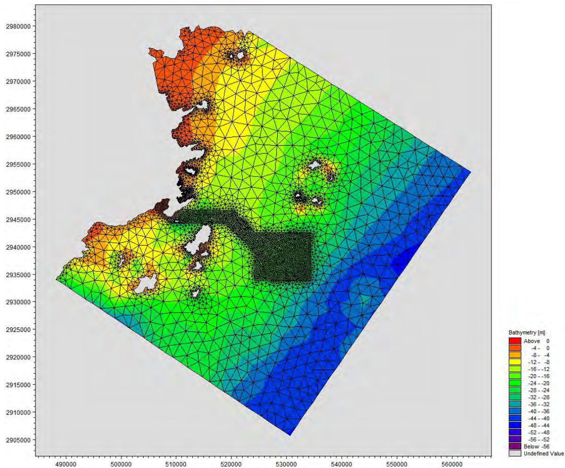
图 5.1-1 模型网格分布及水深图
