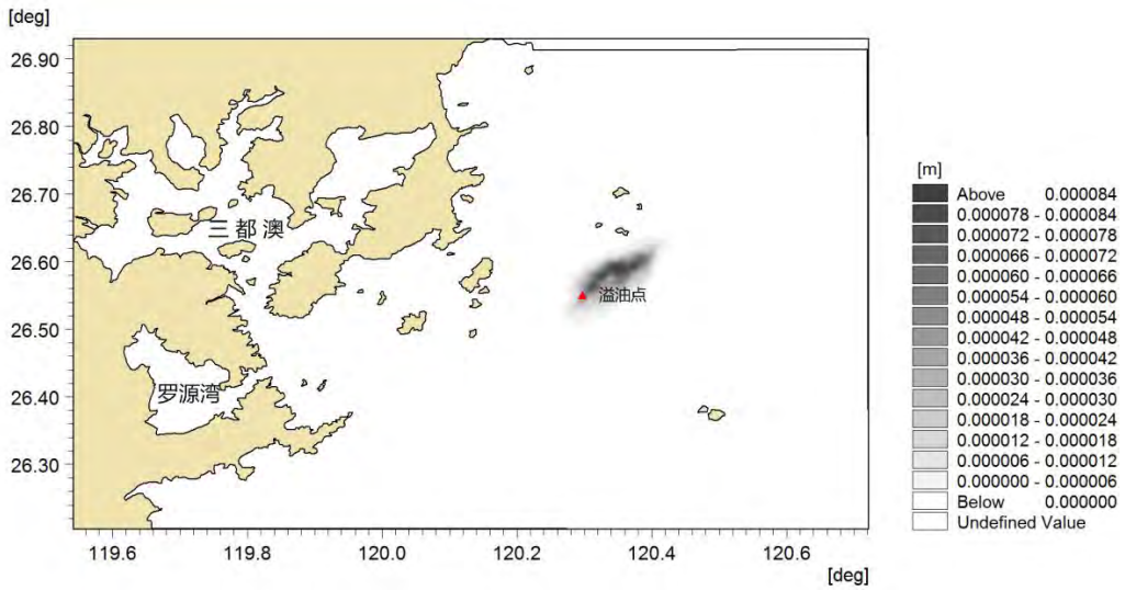
图 6.2-6 SE 高潮时溢油发生 72h 内最大影响范围图（单位：油膜厚度 m）
