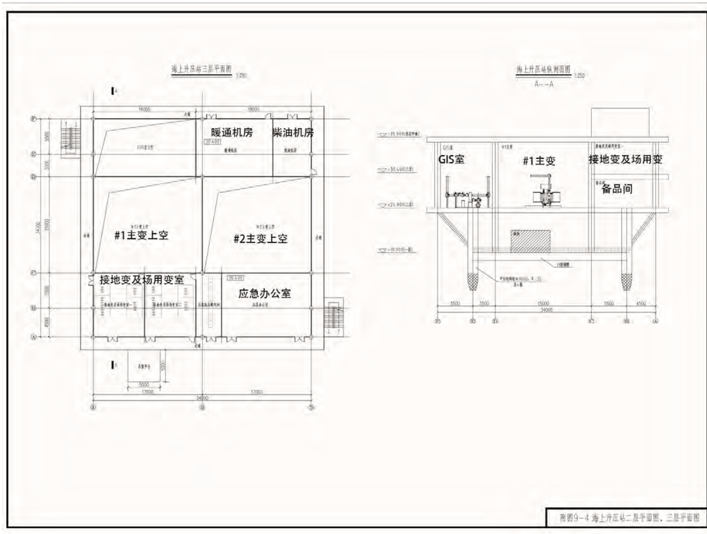
图 3.1-8 海上升压站三层平面及升压站纵剖面图
