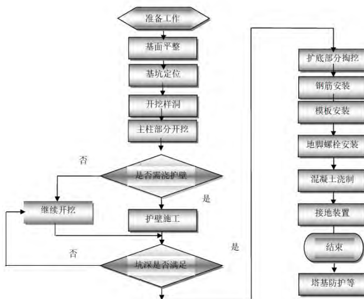
图 3.1-12 基础施工工艺流程图
