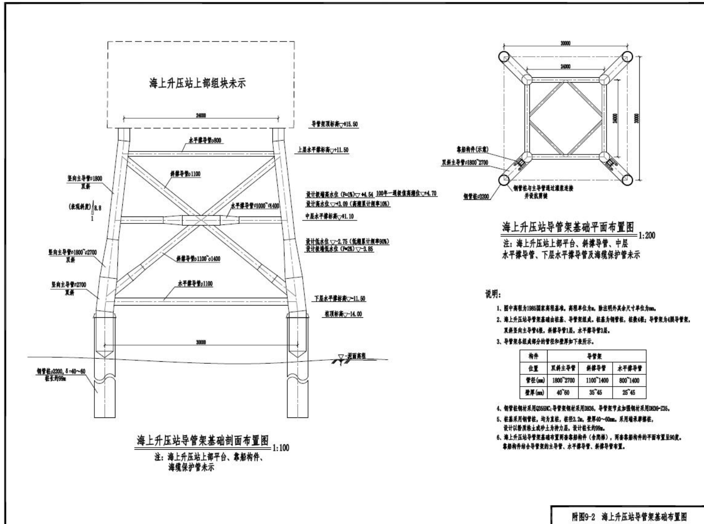
图 3.1-6 升压站基础剖面图
