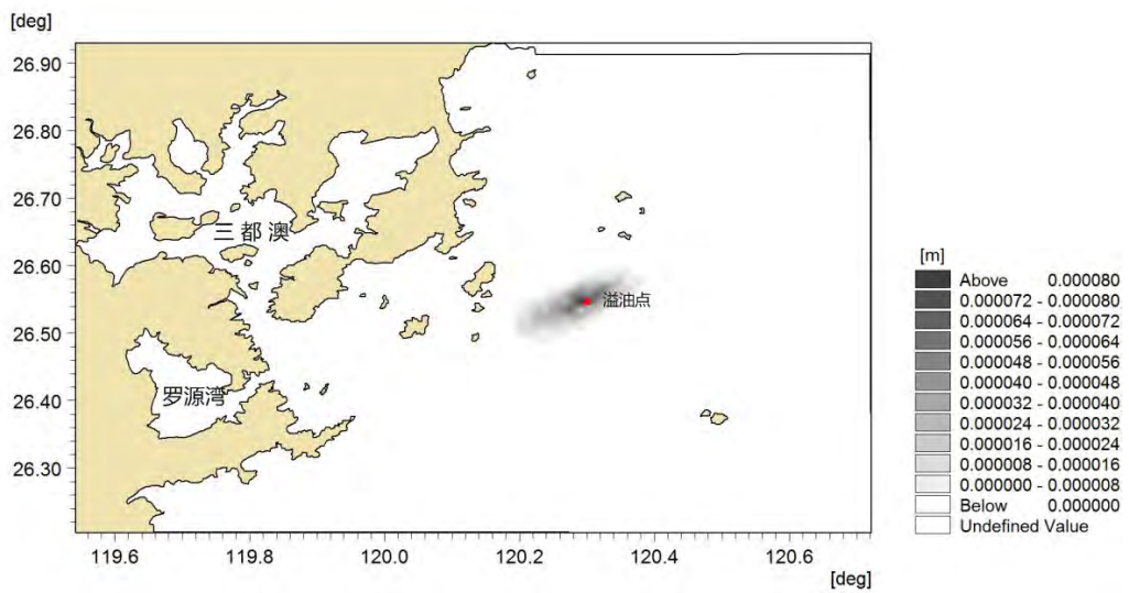
图 6.2-7 SSW 低潮时溢油发生 72h 内最大影响范围图（单位：油膜厚度 m）
