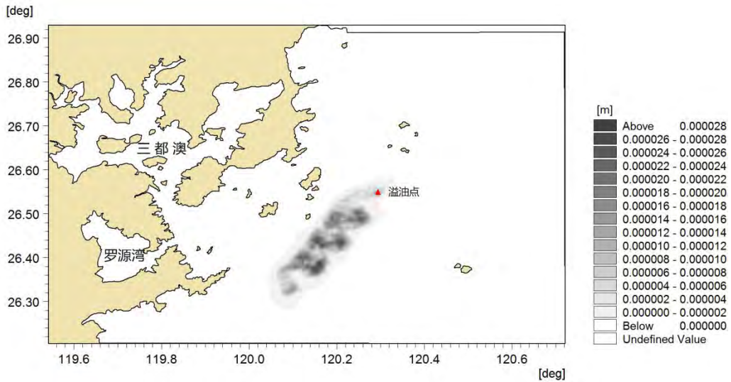
图 6.2-3 NNE 低潮时溢油发生 72h 内最大影响范围图（单位：油膜厚度 m）
