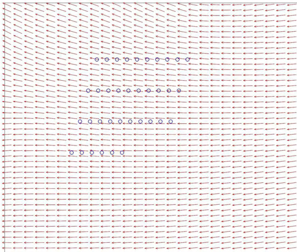
图 5.1-16 大潮期风电场附近海域涨急时刻潮流场变化图 (黑色流矢：工程前；红色流矢：工程后)
