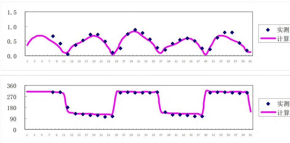
图5.1-9 V6测站流速流向验证图
