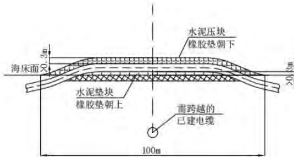
图 3.1-11 海缆交越段施工立面图
