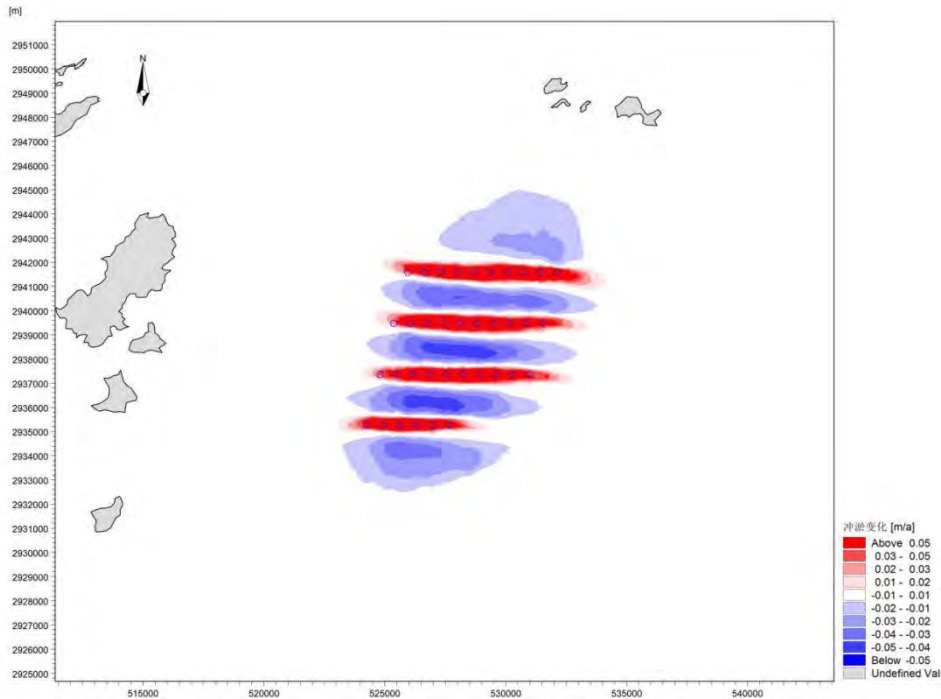
图 5.1-21 风电场建成后年冲淤变化图（单位：m/a） （负值代表冲刷，正值代表淤积）
