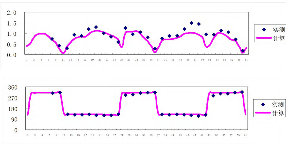
图 5.1-5 V2 测站流速流向验证图
