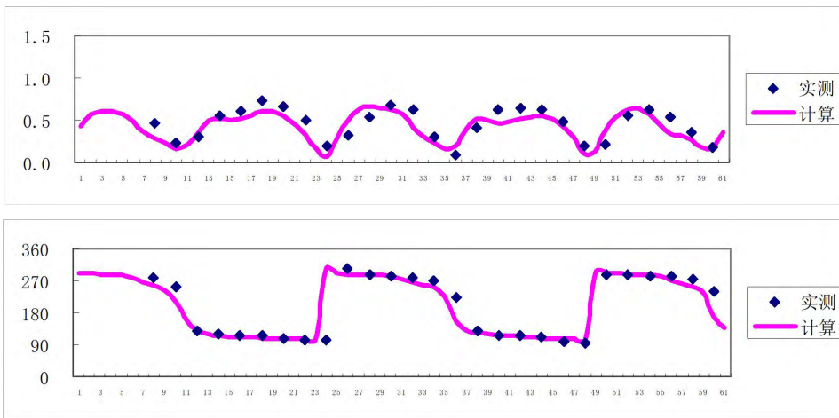
图5.1-8 V5测站流速流向验证图
