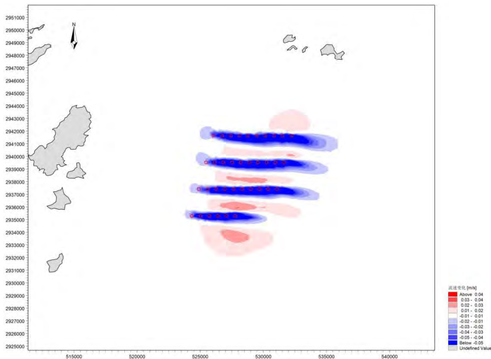
图 5.1-19 工程前后大潮落急流速变化 (单位: m/s)
