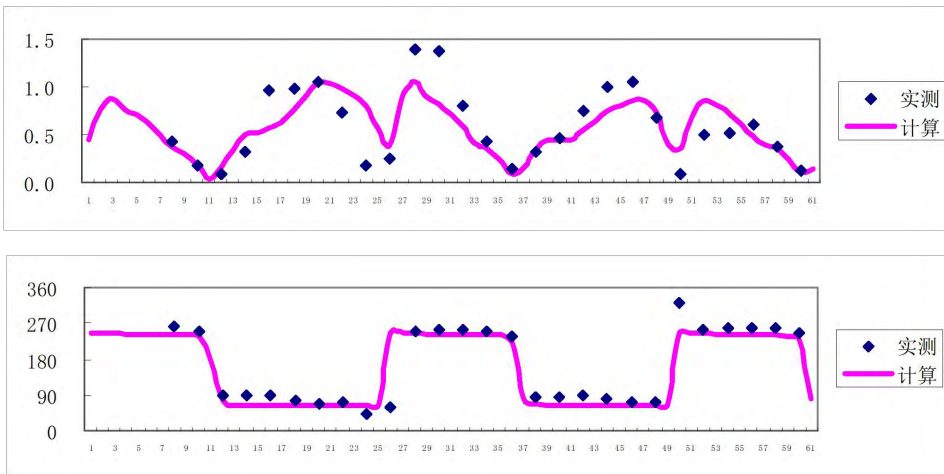
图5.1-6 V3测站流速流向验证图
