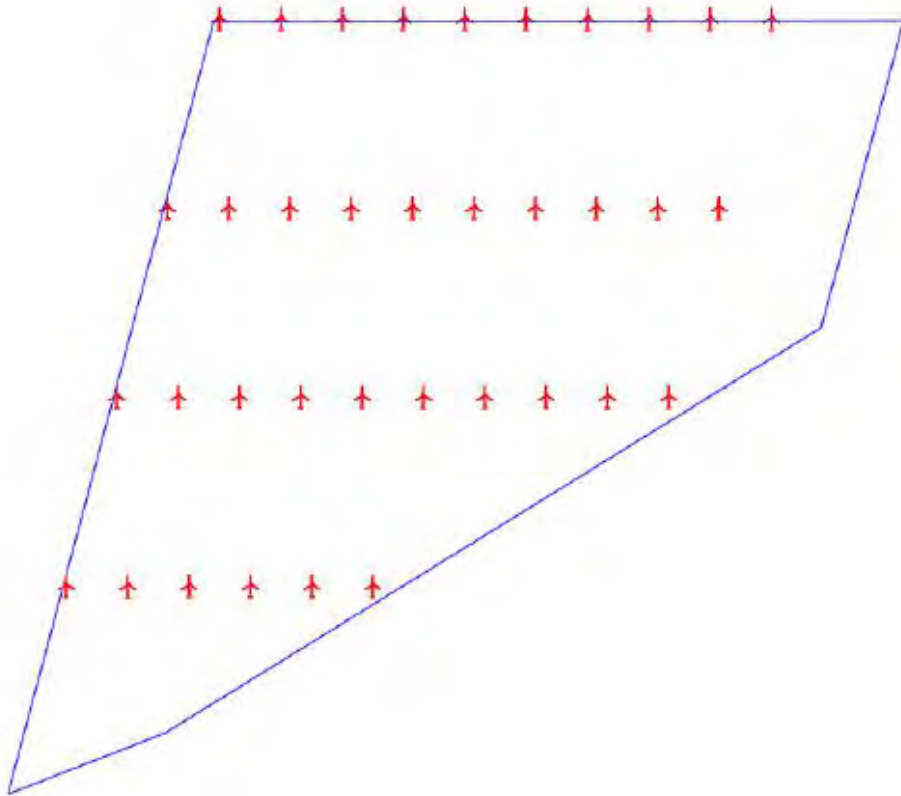
图 3.5-1 宁德霞浦海上风电场工程 B 区布置方案（方案一）
