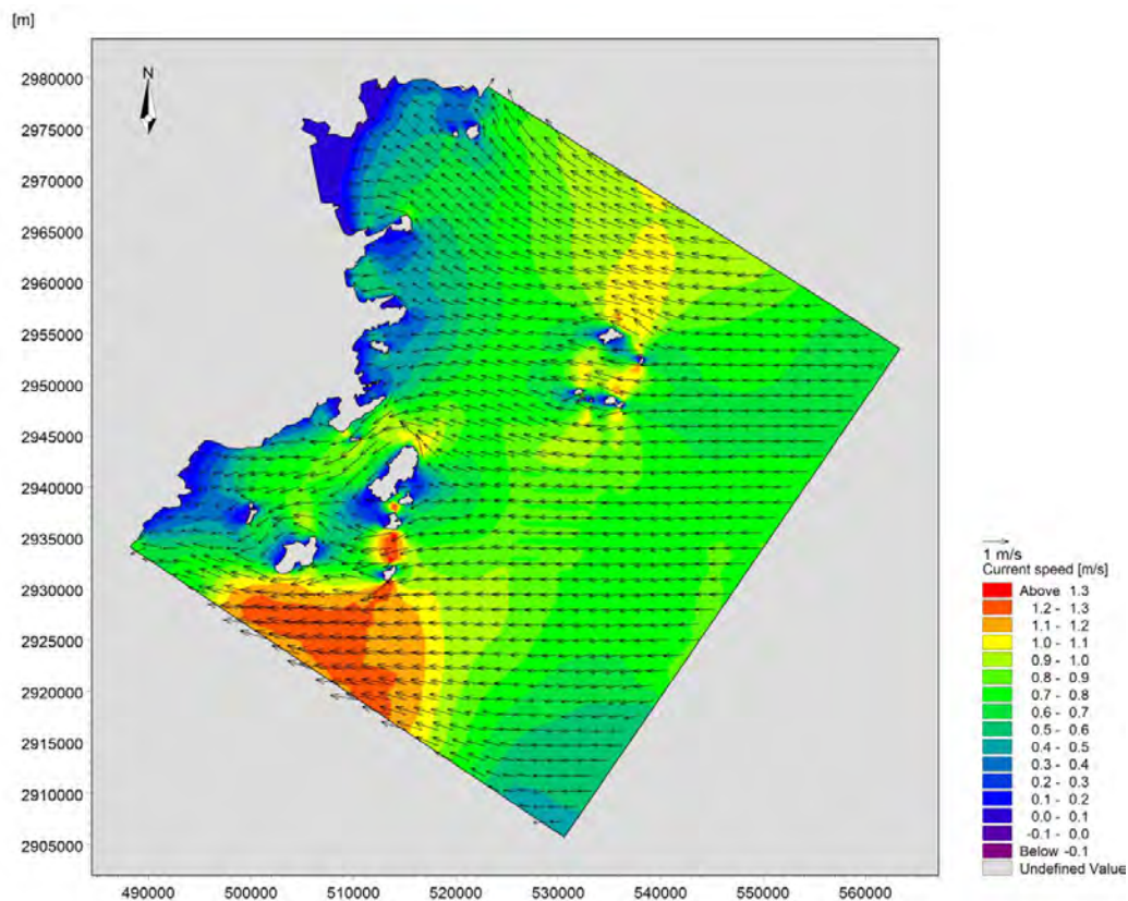
图 5.1-14 大潮期工程附近海域涨急时刻潮流场（工程后）
