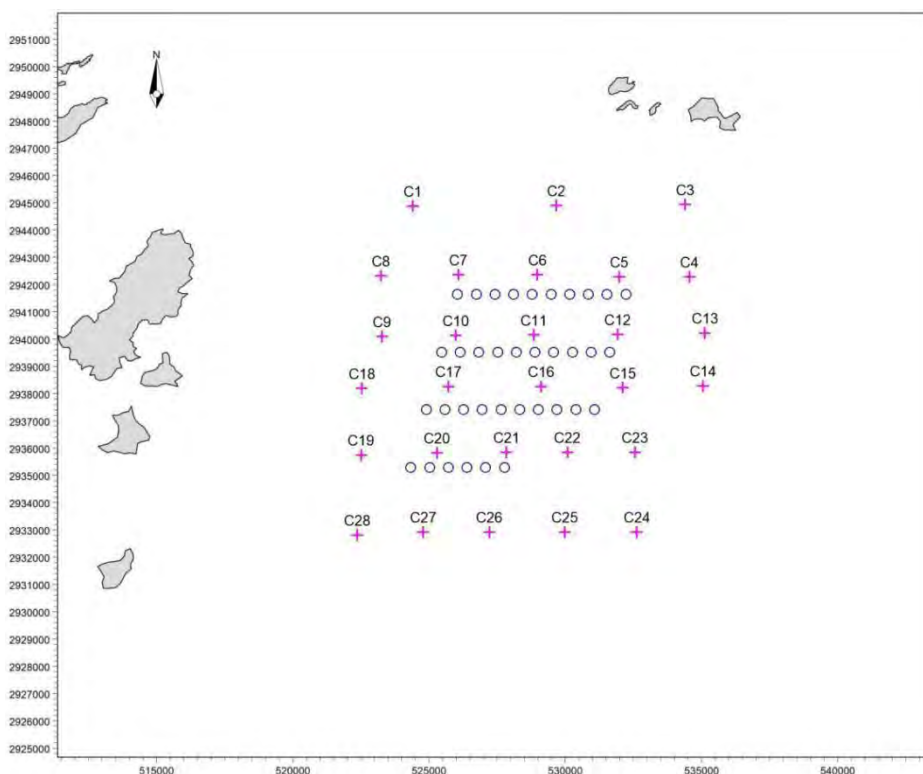
图 5.1-20 工程前后流速变化分析特征点位置
