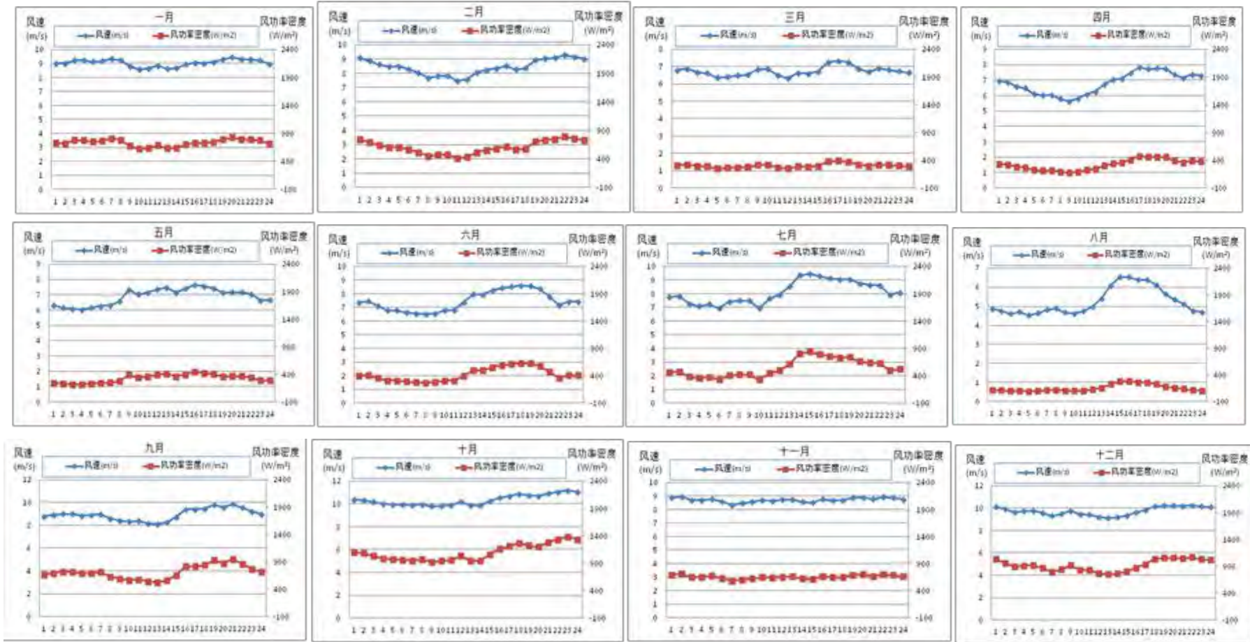
图 4.2-5 测风塔 80m 高度各月逐时平均风速及风功率密度变化曲线
