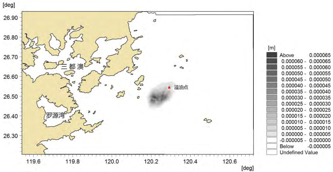
图 6.2-1 静风低潮时溢油发生 72h 内最大影响范围图（单位：油膜厚度 m）
