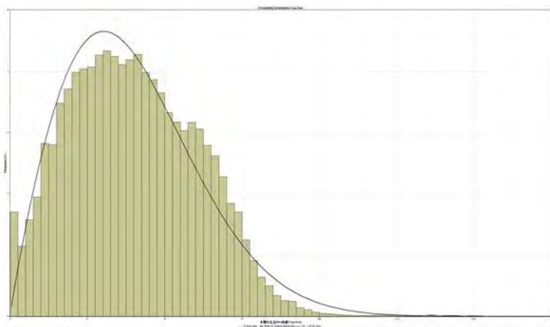
图 4.2-6 测风塔 80m 高度风速频率分布直方图
