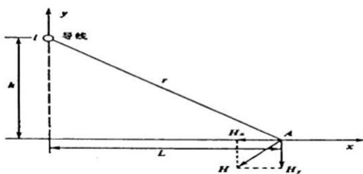
图 5.8-3 磁场向量图
