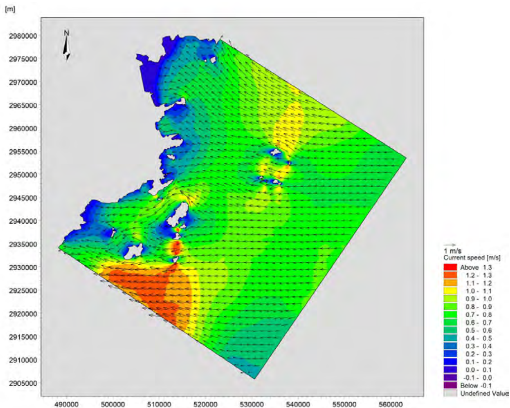
图 5.1-11 大潮期计算海域涨急时刻潮流场（工程前）
