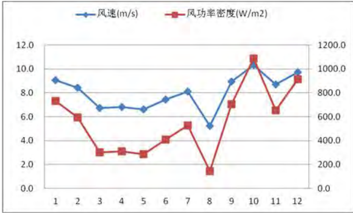
图 4.2-3 测风塔 80m 高度逐月平均风速及风功率密度曲线
