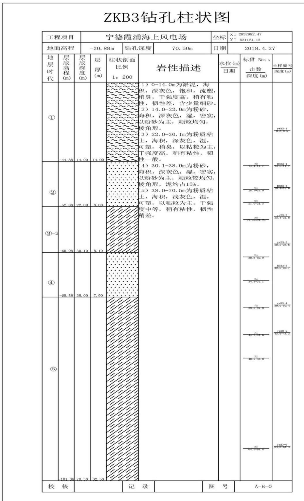
图 4.1-5 ZKB3 钻孔柱状图
