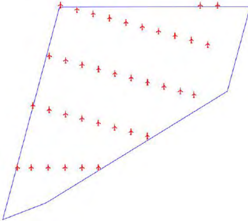
图 3.5-3 宁德霞浦海上风电场工程 B 区布置方案（方案三）
