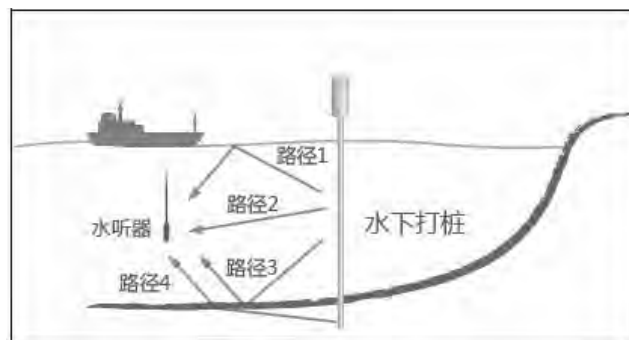
图 5.7-1 水下打桩噪声传播路径
