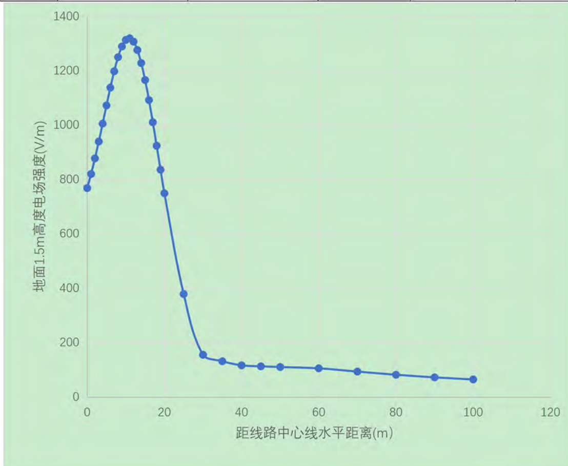
图 5.8-5 线路电场强度变化趋势图
