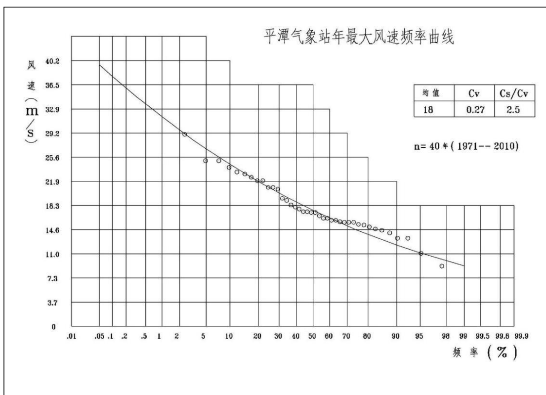
图 4.2-10 平潭气象站最大风速频率曲线图
