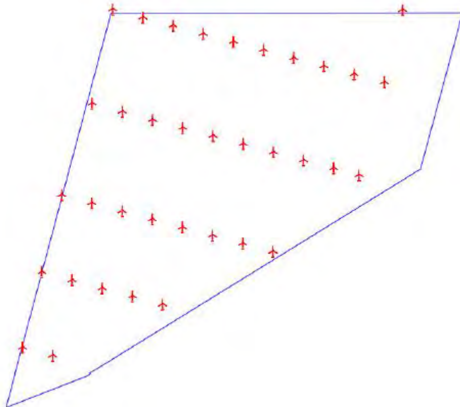
图 3.5-2 宁德霞浦海上风电场工程 B 区布置方案（方案二）
