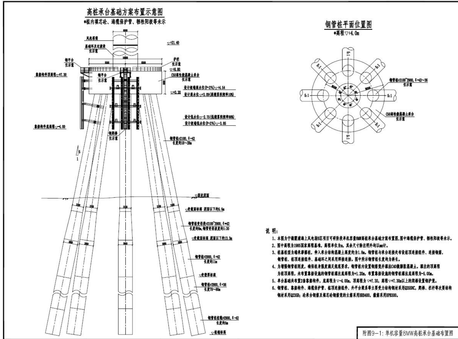
图 3.1-5 风机基础立面图
