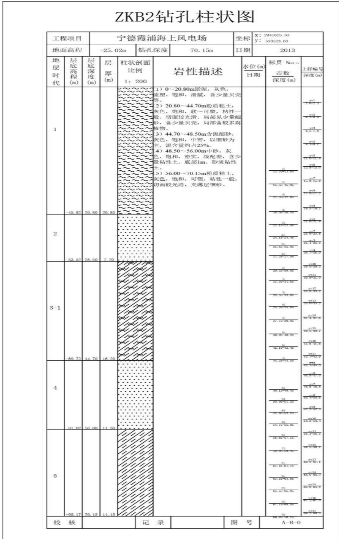
图 4.1-4 ZKB2 钻孔柱状图
