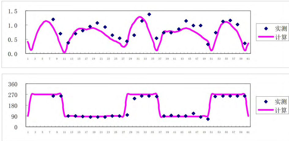
图 5.1-4 V1 测站流速流向验证图
