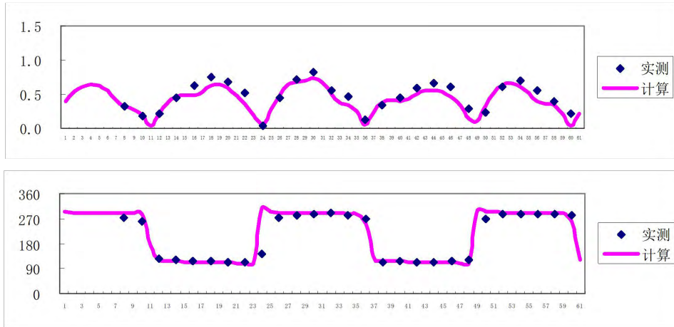
图5.1-7 V4测站流速流向验证图
