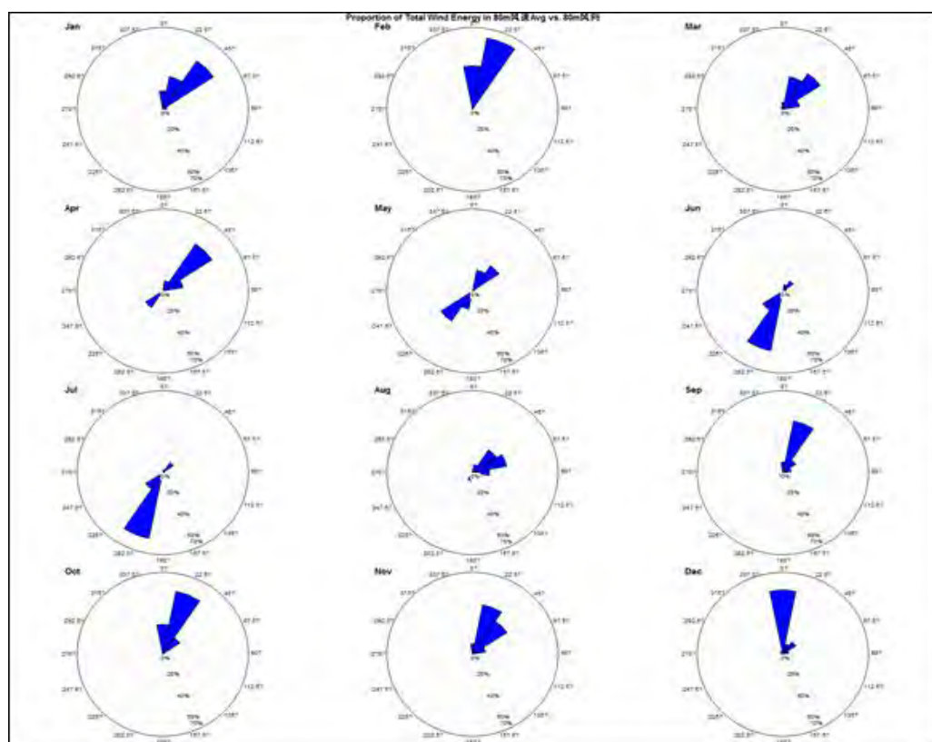
图 4.2-9 测风塔 80m 高度各月风能频率玫瑰图
