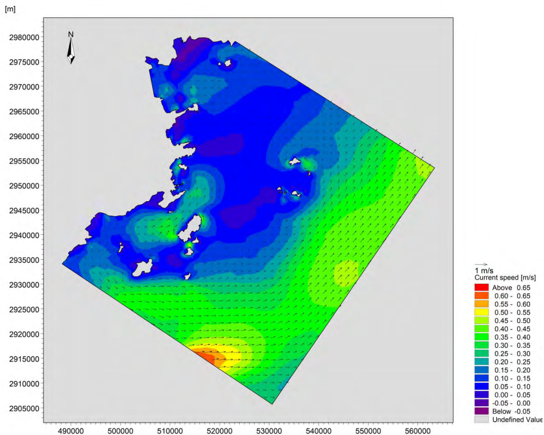
图 5.1-10 大潮期计算海域低潮时刻潮流场（工程前）
