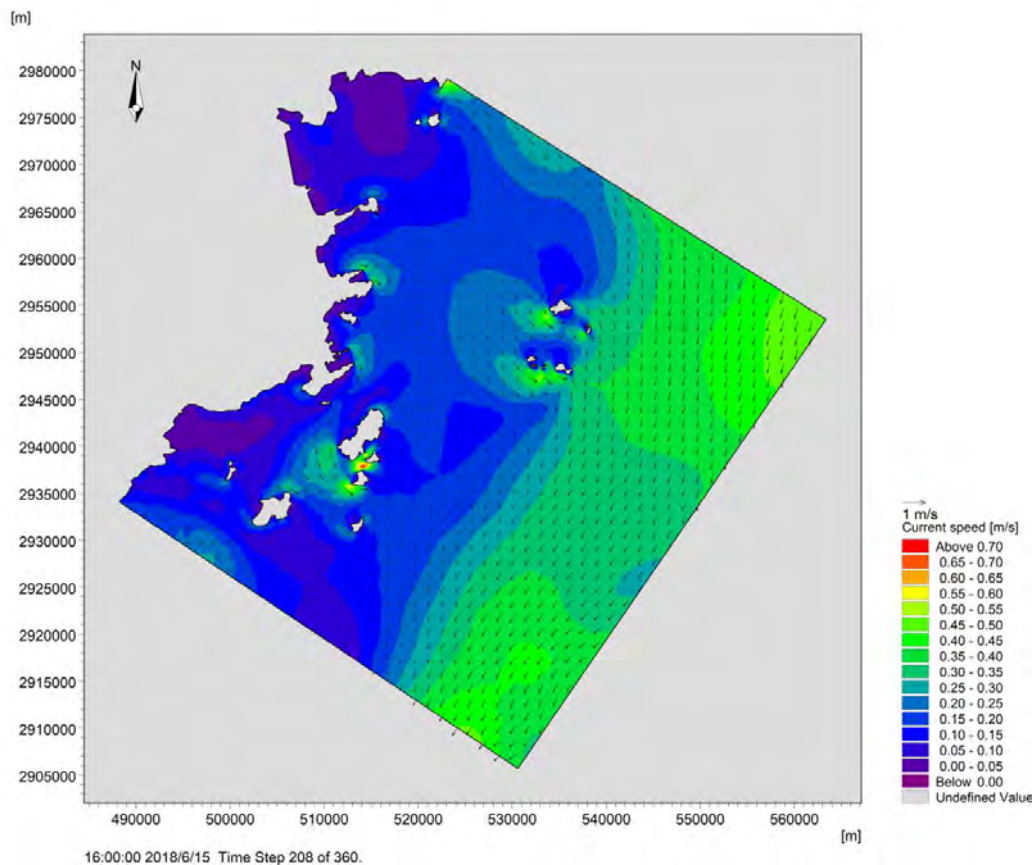
图 5.1-12 大潮期计算海域高潮时刻潮流场（工程前）
