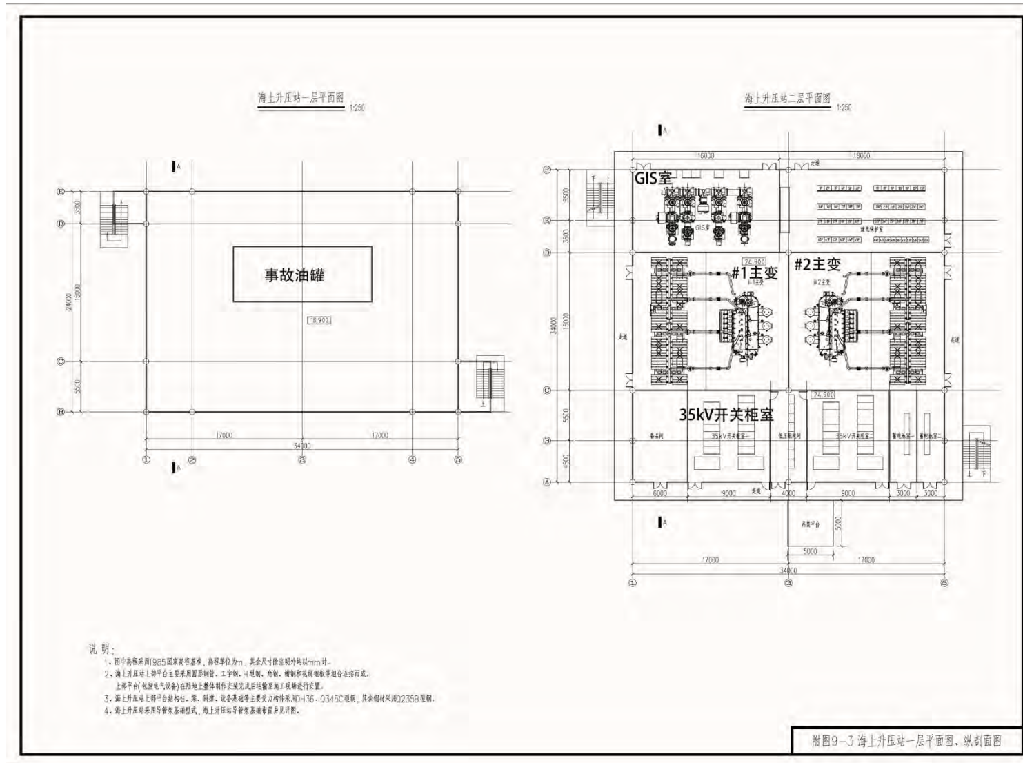
图 3.1-7 海上升压站一、二层平面图
