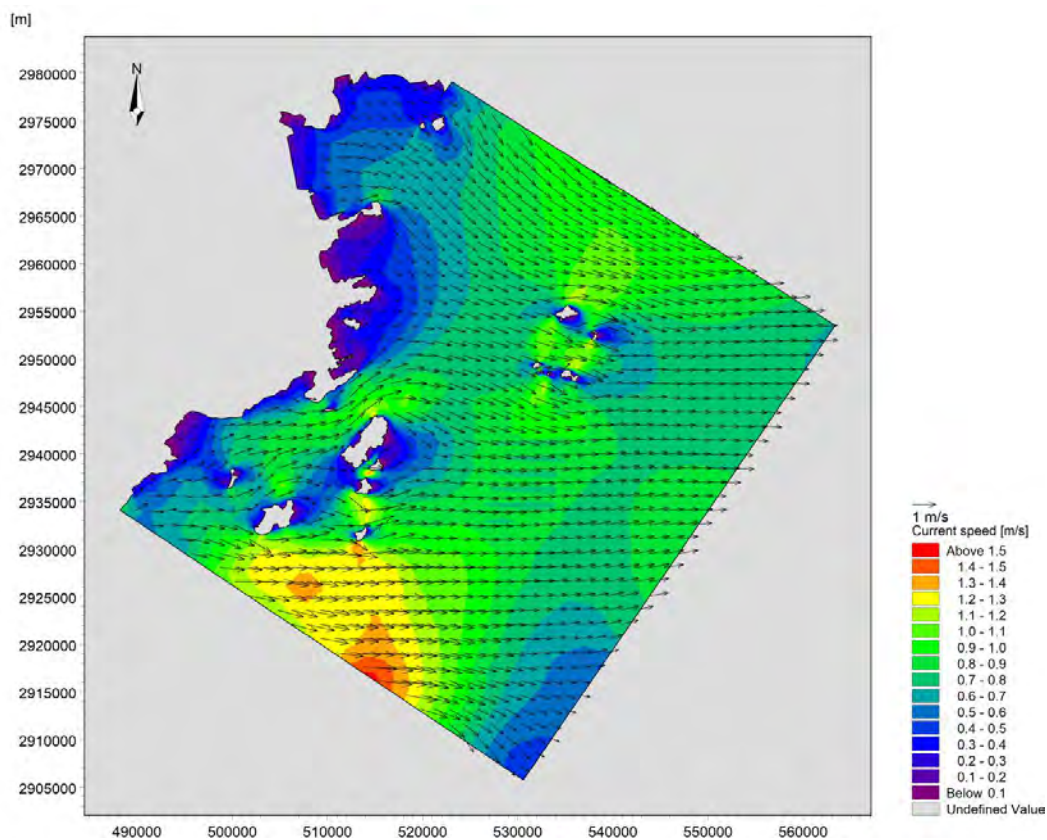
图 5.1-15 大潮期工程附近海域落急时刻潮流场（工程后）
